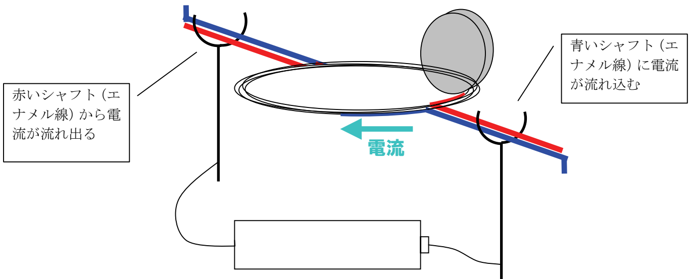
図 3-1 完全な整流子を備えるモータの原理図 (一つの状態)
