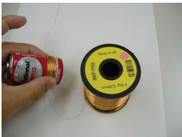
写真 3 コイル製作
