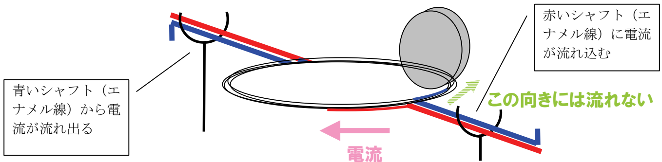
図 3-2 完全な整流子を備えるモータの原理図 (図 3-1 から電機子がひっくり返った)
