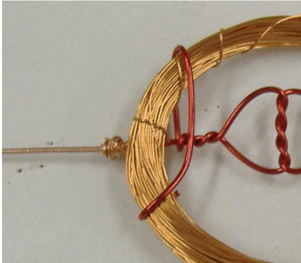
写真 2-13 シャフトとコイルの接続部
