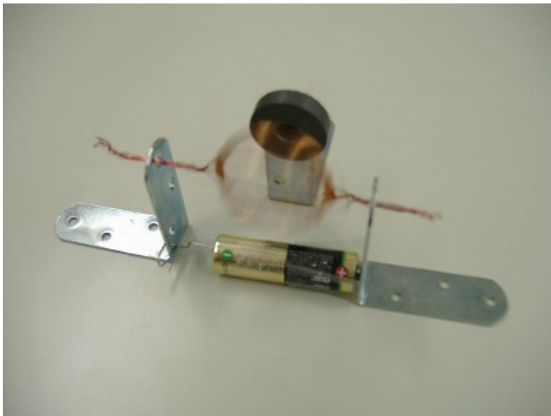
写真 3-2 完成したモータ
